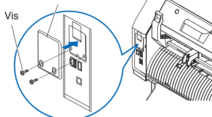
Couvercle du module du réseau local sans fil
