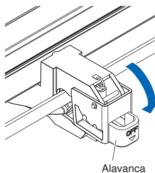
Alavanca
