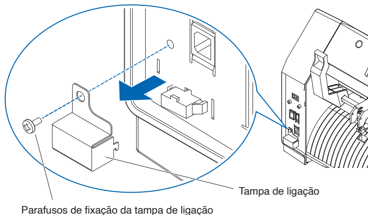
Parafusos de fixação da tampa de ligação
